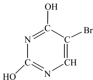
5-Бромурацил
