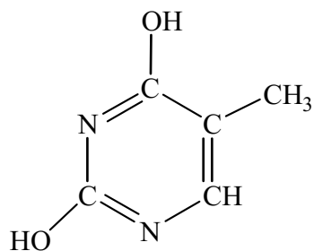
Тимин (5-метилурацил)
